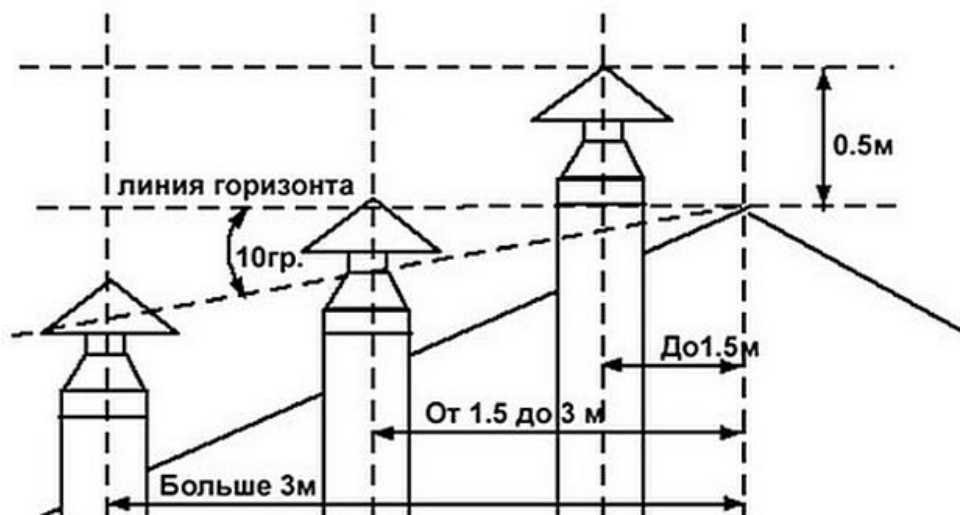
Рисунок 10 — Схема размещения дымоходов.
